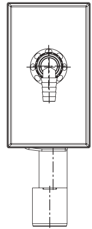
Waschgerätesiphon nur Ablaufanschluss
